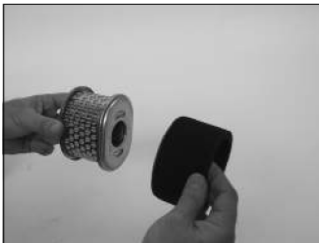
5) Осторожно извлечь фильтр грубой очистки и очистить пластинки
